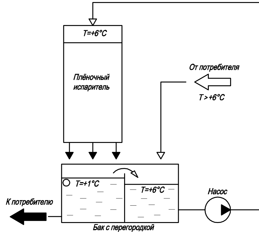
Двухконтурная схема
