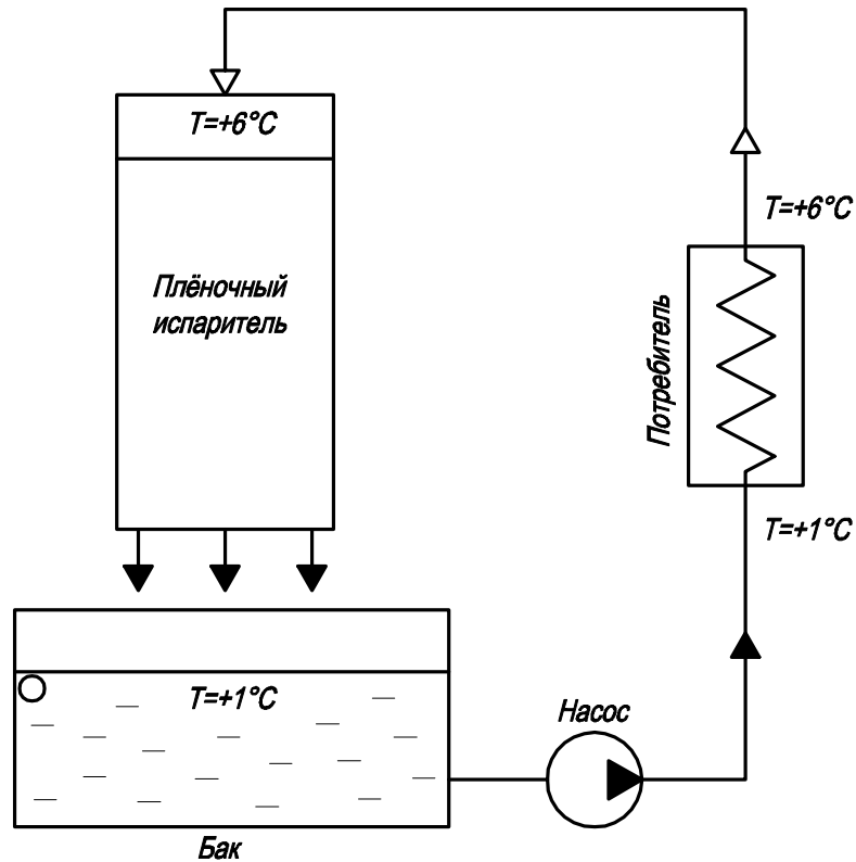
Одноконтурная схема
